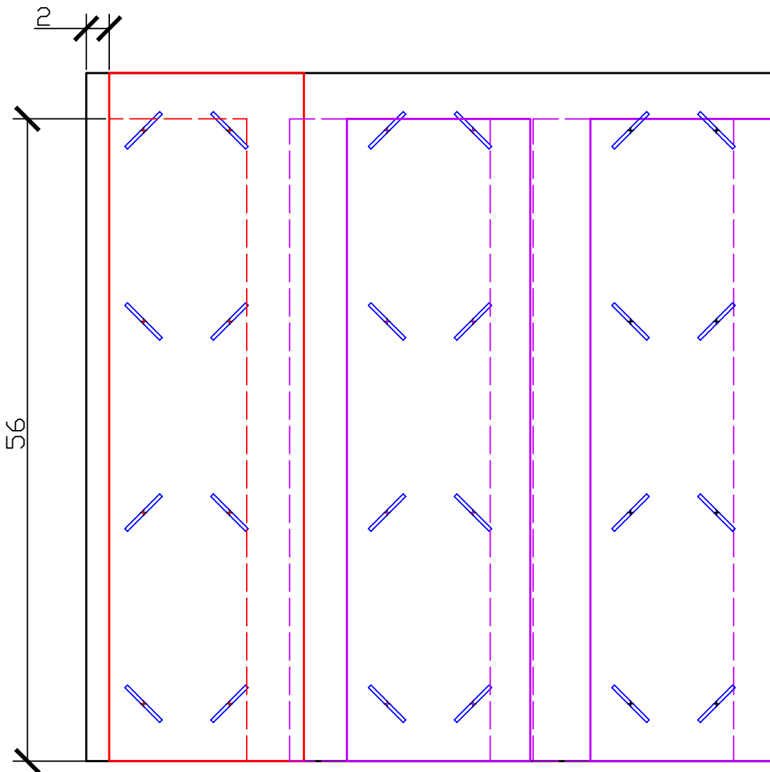
7,5-es osztású dupla panel
